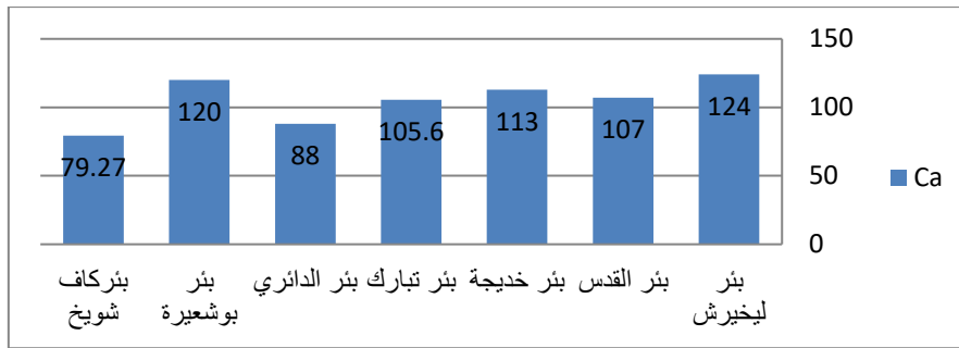
شكل(6): قيم الكالسيوم Ca للآبار في منطقة الدراسة (مليغرام/ لتر)
