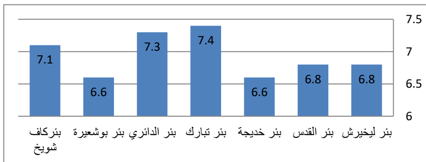
شكل (2) قيم الرقم الهيدروجيني pH للآبار في منطقة الدراسة
