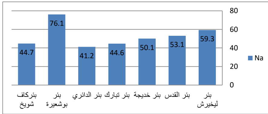
شكل (8): قيم الصوديوم Na للأبار في منطقة الدراسة (مليغرام /لتر)
