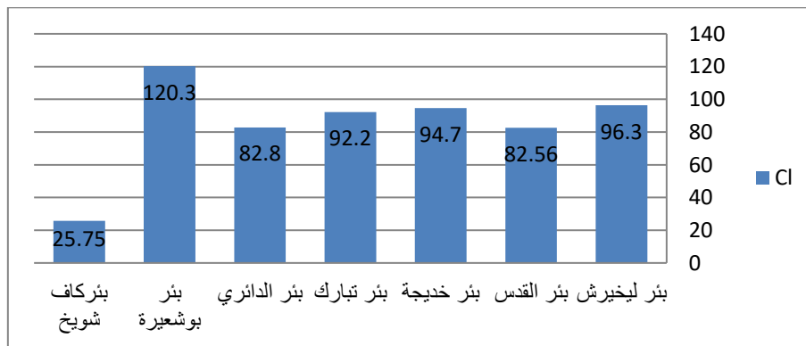
شكل (10): قيم الكلوريد Cl للآبار في منطقة الدراسة (مليغرام/ لتر)
