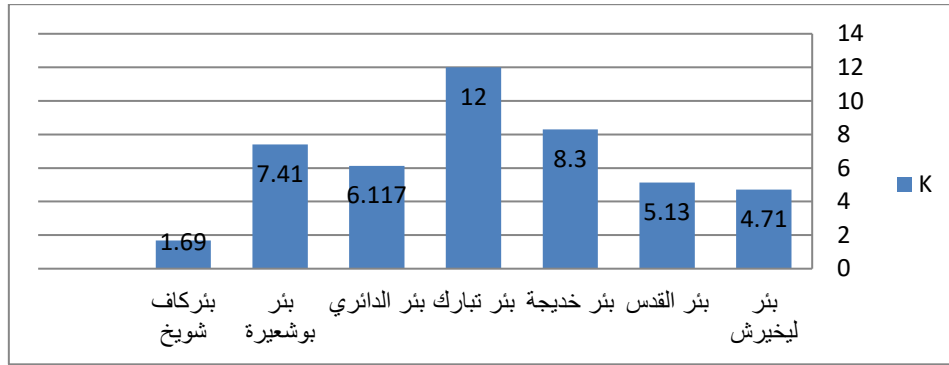
شكل (9): البوتاسيوم k للآبار في المناطق المدروسة (مليغرام/ لتر)
