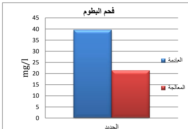
الشكل (2) تأثير فحم البطوم علي تنقية عنصر الحديد في المياه العامة
