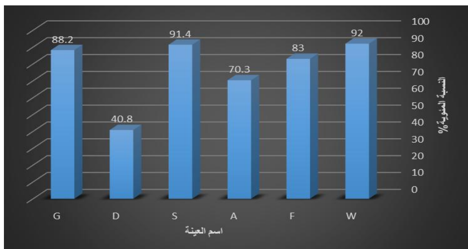
الشكل 1 كفاءة تنقية الاملاح الذائبة الكلية %
